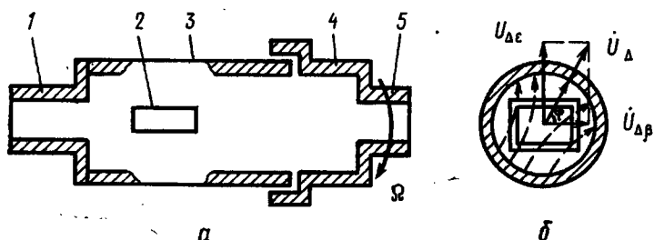
Рис. 2.23. Волноводный модулятор а — конструкция; б — суммирование сигналов в круглом волноводе; 1 — вход u_{\Delta \beta} ; 2 — вход u_{\Delta \epsilon} ; 3 — круглый волновод; 4 — вращающаяся часть; 5 — прямоугольный волновод
