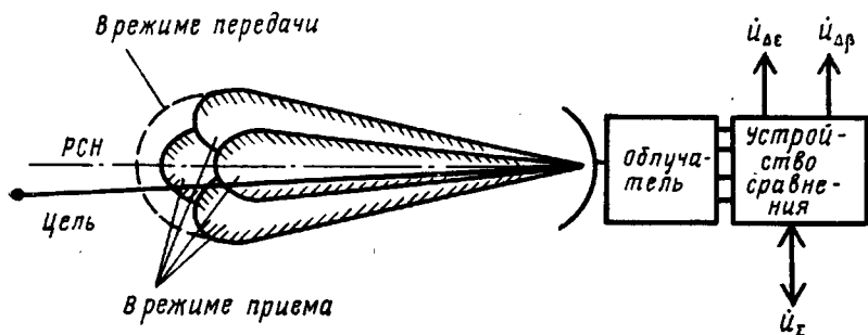
• Рис. 2.20. Диаграмма направленности антенны ССЦ
