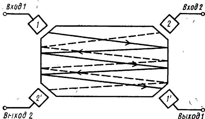
Рис. 2.10. Двухканальная УЛЗ:
