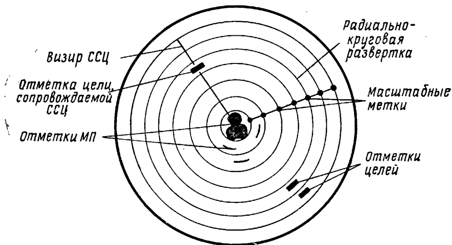
Рис. 2.3. Вид экрана ИКО
