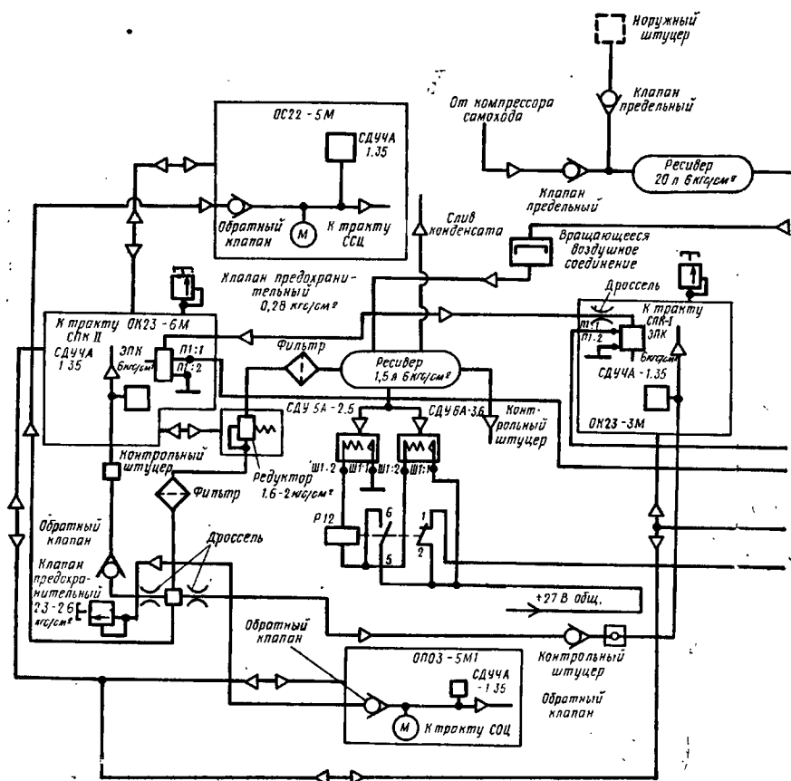
Рис. 2.63. Схема пневмосисте
