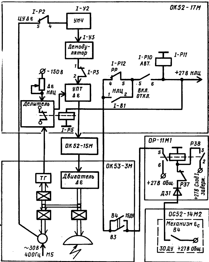
Рис. 2.43. Упрощенная функциональная схема СУА СВР в режиме НЛЦ
