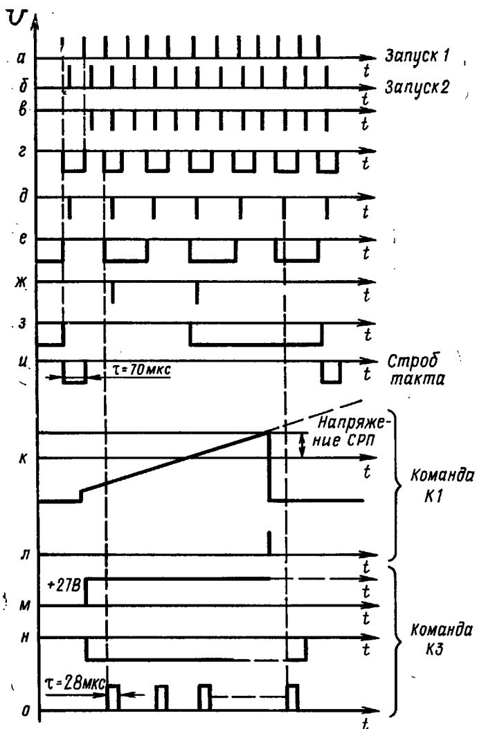
Рис. 2.56. Осциллограммы, поясняющие работу шифратора
