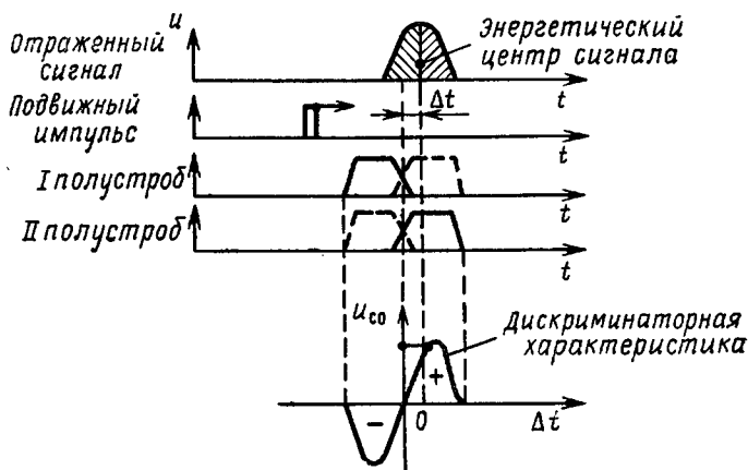
Рис. 2.34. Формирование сигнала ошибки в канале автосопроеждения
