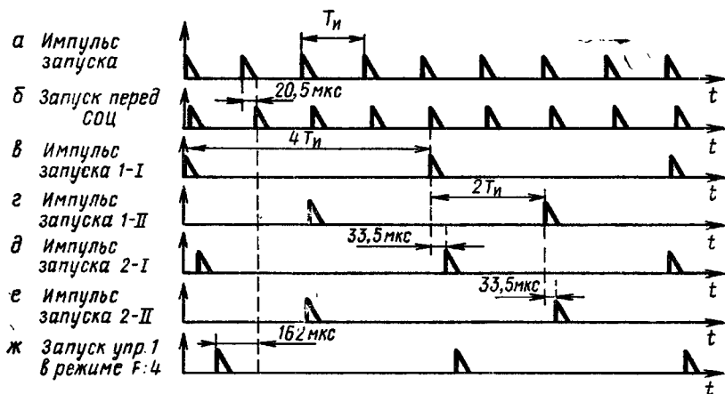
Рис. 2.32. Временные диаграммы схемы формирования запуска СБР и СПК
