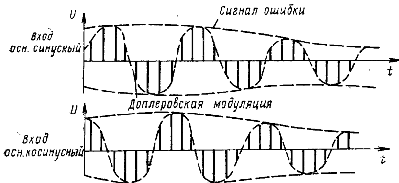
Рис. 2.28. Видеосигналы на входах канала ОЦ блока ОС51-8М
