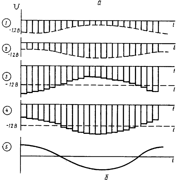
Рис. 2.26. Система ВСО в штатном режиме: а — структурная схема; б — временные диаграммы
