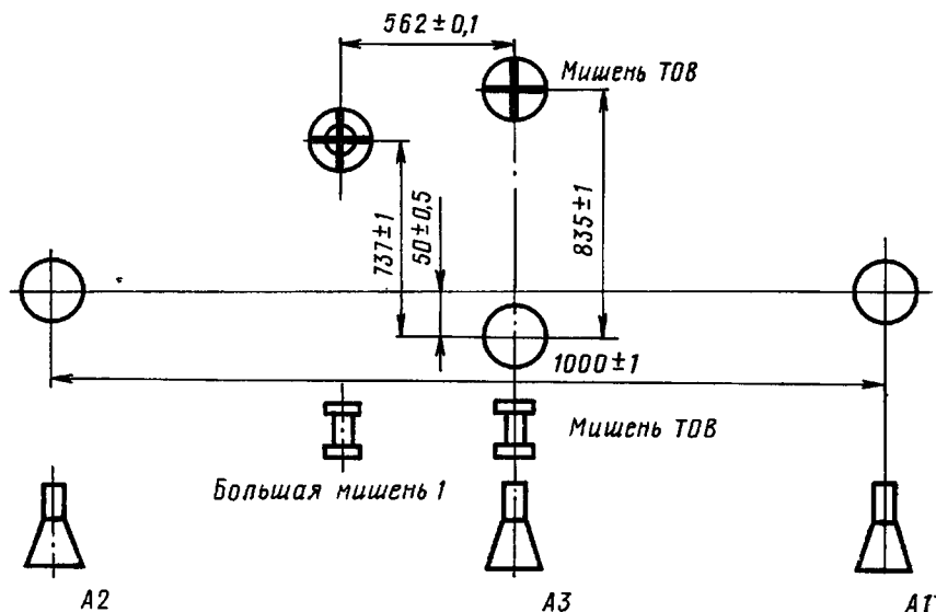
Рис. 4.1. Расположение мишеней и рупорных антенн блока ОЮ07-2
