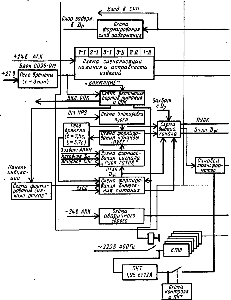
Рис. 2.58. Структурная схема
