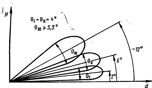
Рис. 2.1. Диаграмма направленности антенны СОЦ
