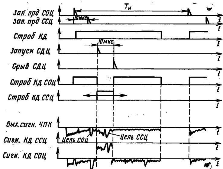
Рис. 2.9. Временные диаграммы узла стробирования
