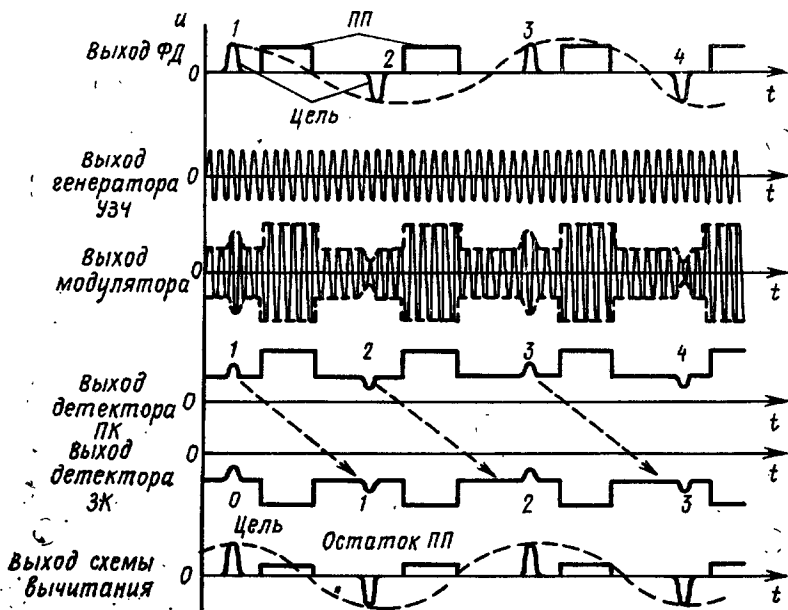
Рис. 2.11. Временные диаграммы канала вычитания \Delta
