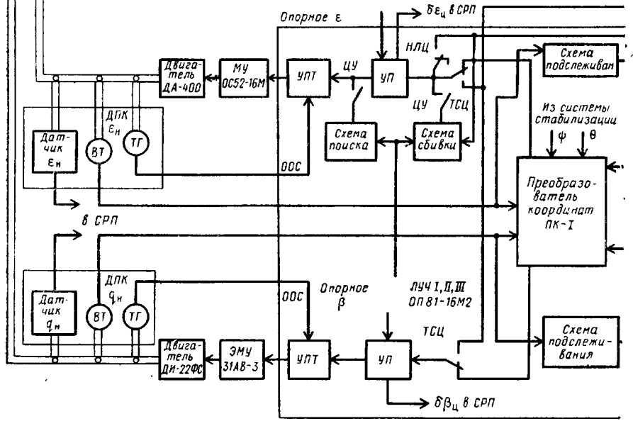
Рис. 2.19. Структур
