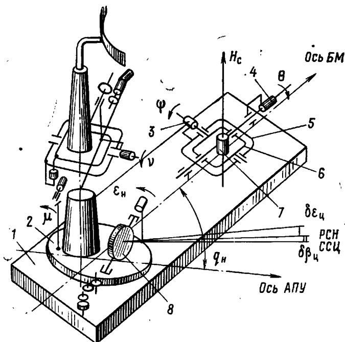
Рис. 2.14. Кинематическая схема системы стабилизации
