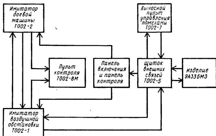
Рис. 4.3. Структурная схема тренажера
