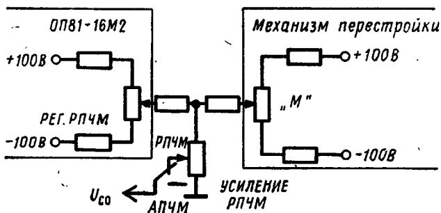
Рис. 2.6. Электрический мост сопротивлений в режиме РЧМ
