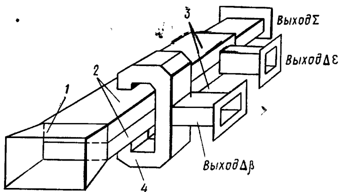
Рис. 2.22. Облучатель с устройством сравнения:
