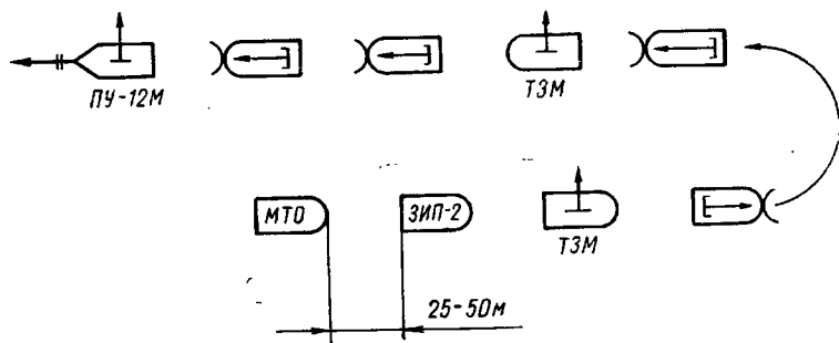
Рис. 6.2. Схема исходного порядка батареи
